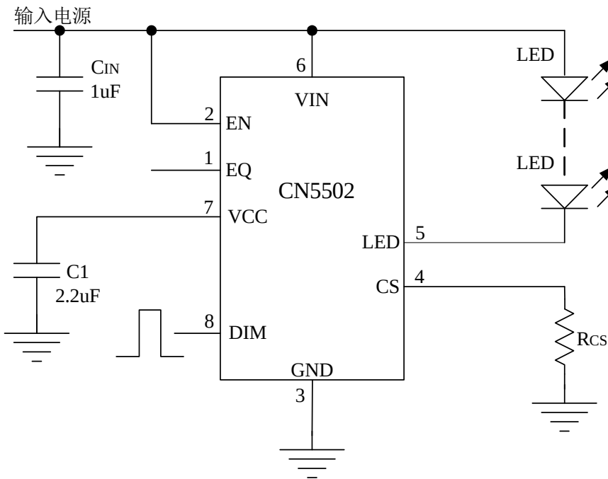
图 2 典型应用电路(PWM 信号调光)
