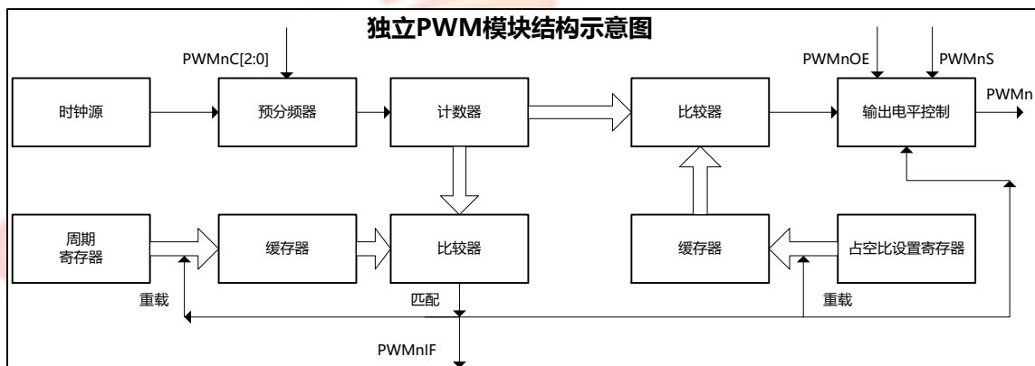
PWM0 结构示意图
