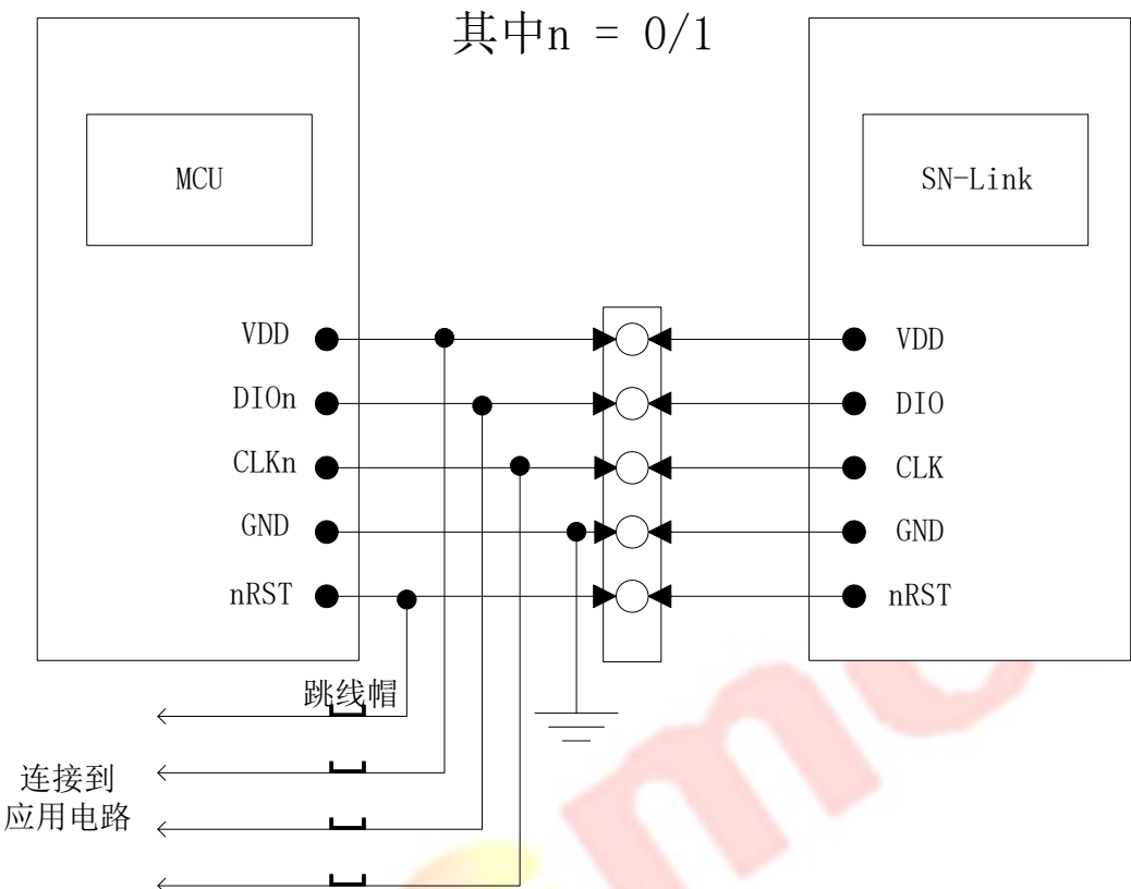
ODC/ICP接口示意图
