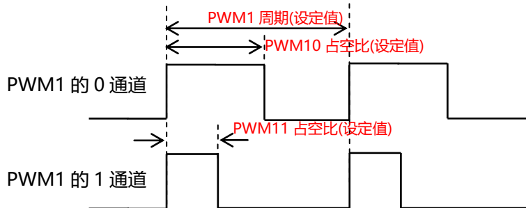
PWM1 独立输出模式 (以 0 和 1 通道为例说明，默认情况下，每个通道的占空比时间表示其输出高电平的时间)
