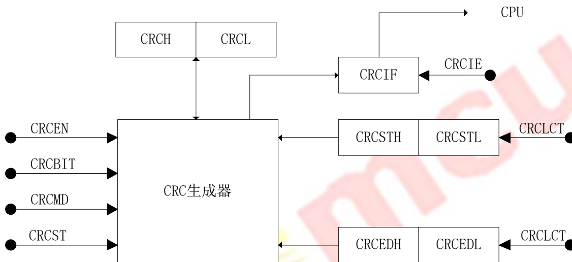
CRC生成器示意图
