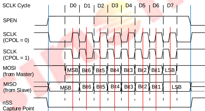
CPHA = 0 时的数据传输示意图
