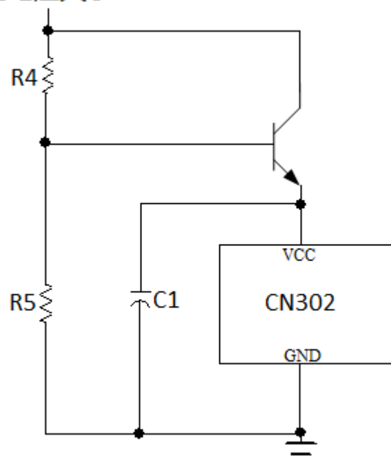
图9 通过电阻分压产生CN302工作电源
