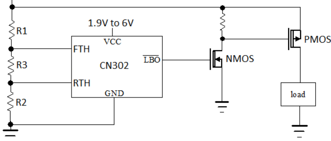
图7 VBAT&gt;6V, CN302控制P沟道场效应晶体管
